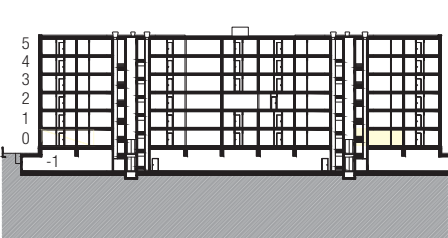
Sezione tipo
