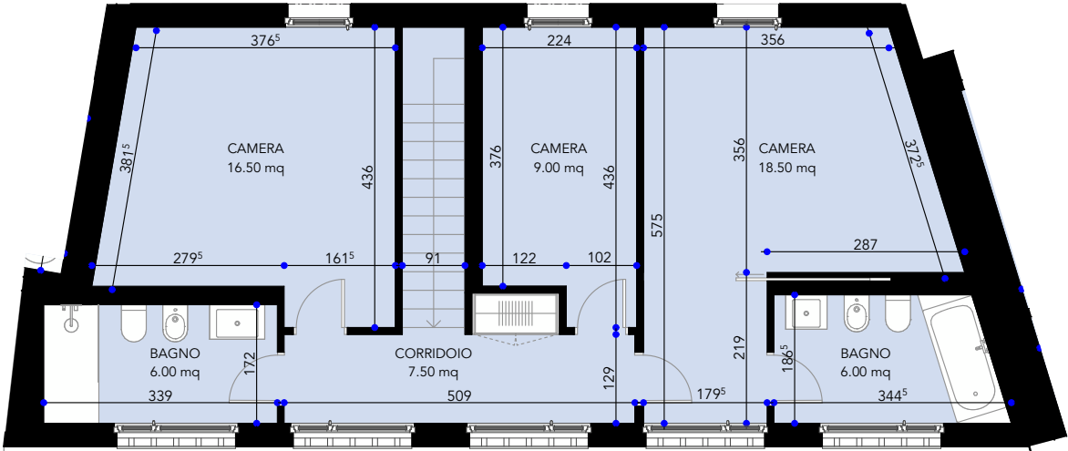
PIANO PRIMO Altezza locali da 2.60 a 3.40
