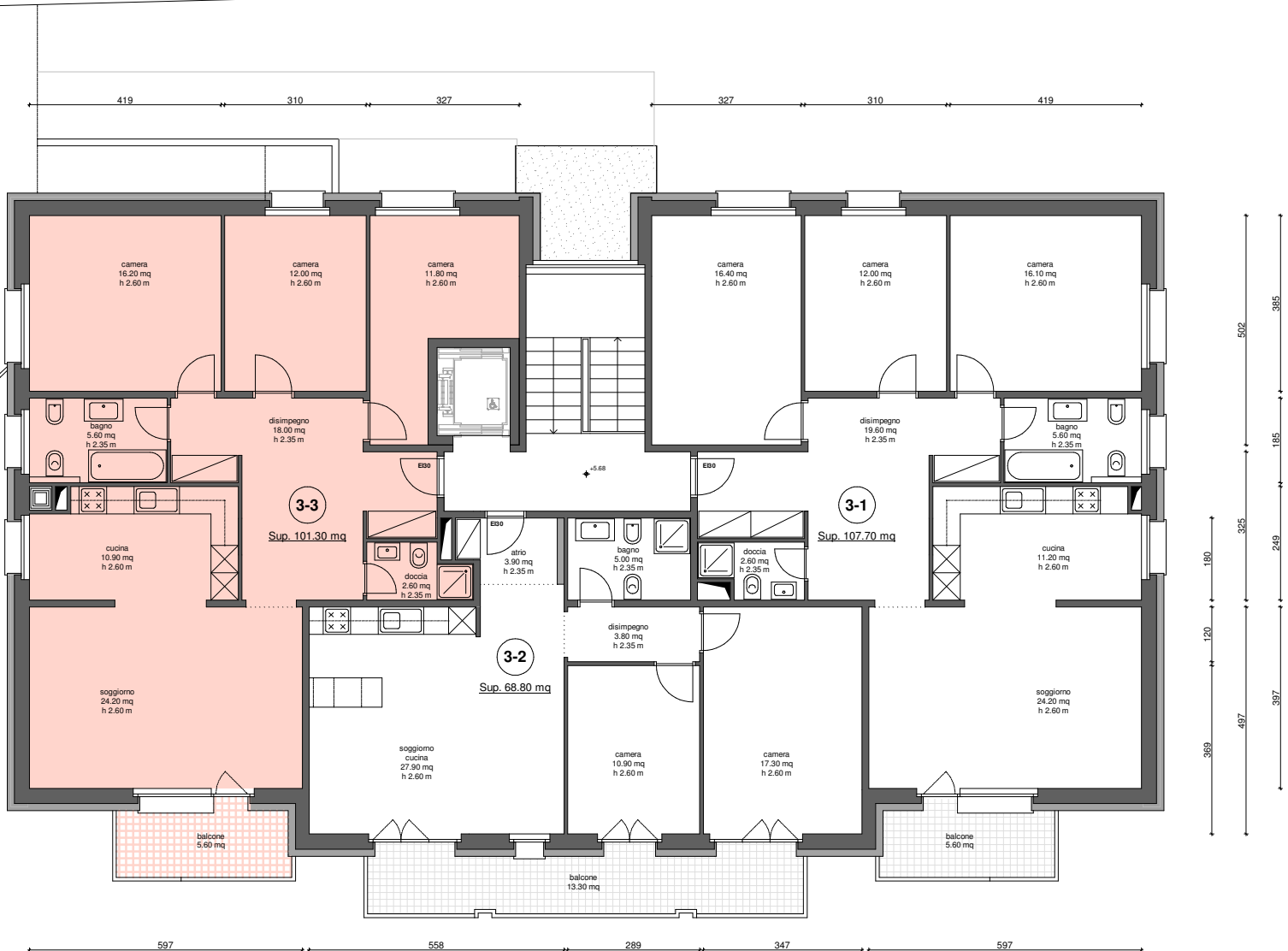
STABILE KUSCO - RIVA SAN VITALE TERZO PIANO
